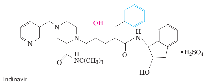
Indinavir
