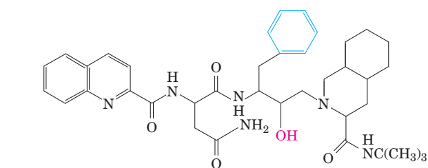
Saquinavir
