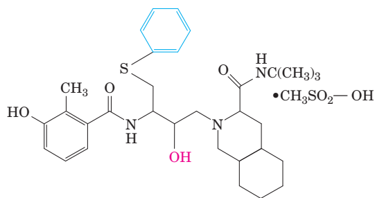
Nelfinavir
