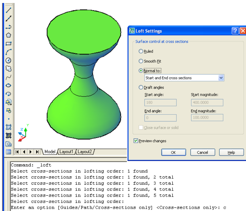
شکل ۸۹-۱) د پوڻلود برابرول او سمول (Loft Settings) د عادي او طبعي سطحي (Normal) انتخاب کي د شروع او اخیرني عرضاني قطعه (Start and End cross section) ٽاڪلو
