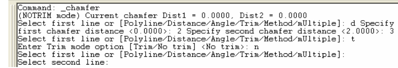
شکل د (۴۰-۲) Chamfer) کپنه چي (no trim) وي
