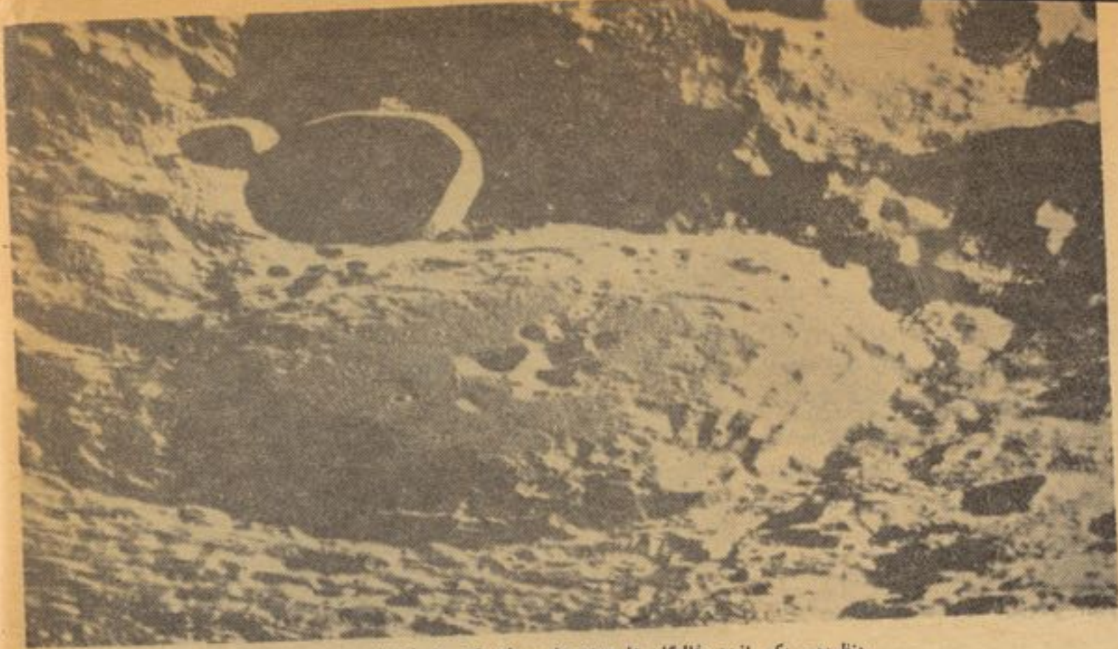
منظره‌یی یکی ازین خالیگاه ها ووادی‌های سطح قمر از نزدیک
