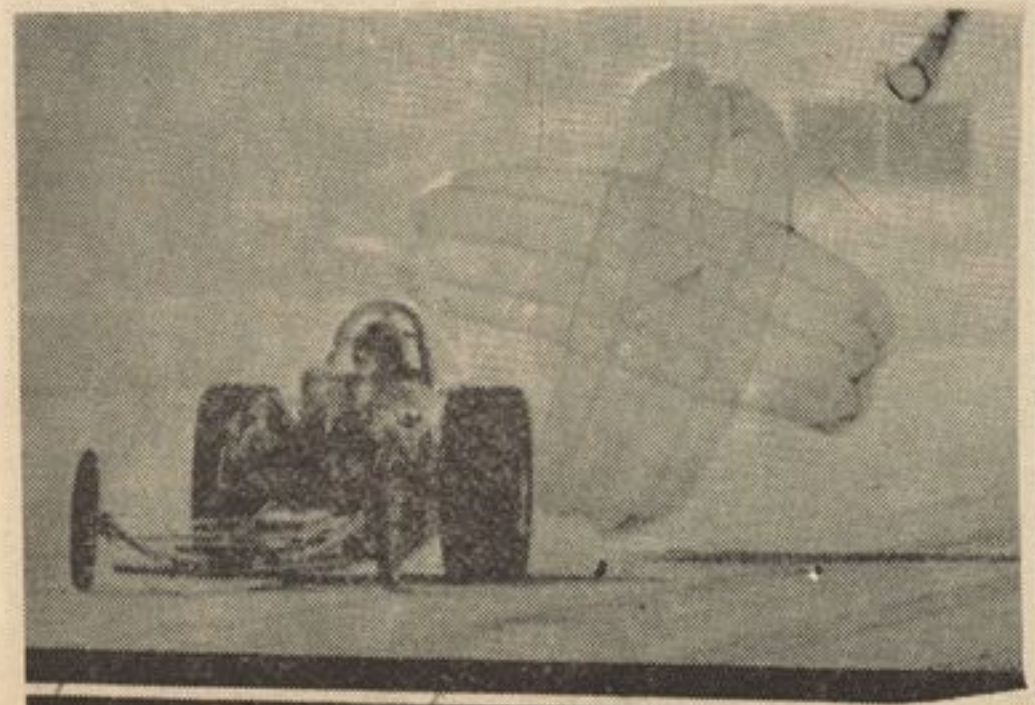
پارا شوت مخصوص كه در عقب موتر قرار دارد در توقف دادن موتر كمك ميكند .
