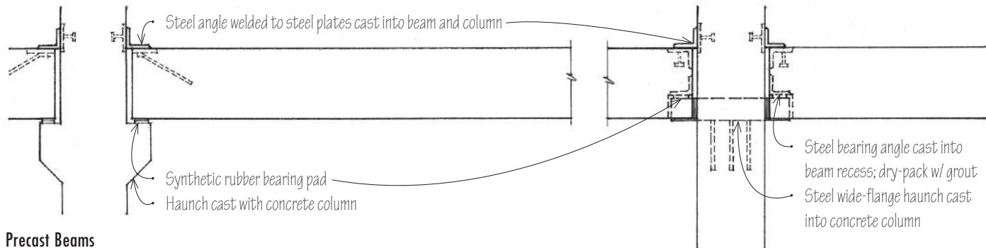
Precast Beams
