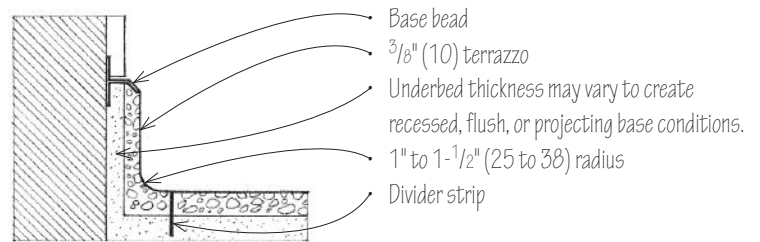
Terrazzo Base
