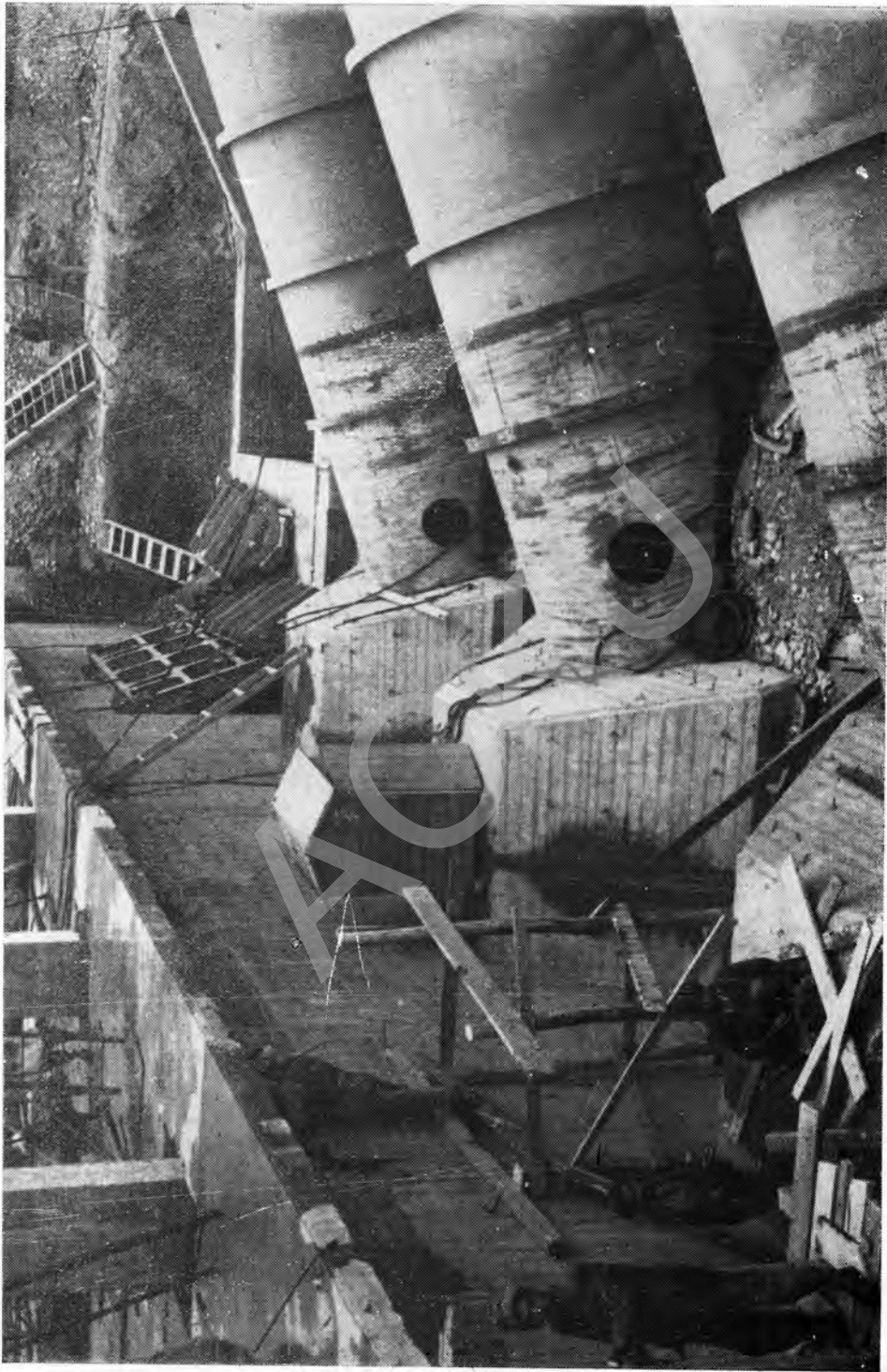
په قطن كښې ددهنه غوري دبرېښا، دافبريكي داوبو لگولو ټولونه چه ددې ټولنو پواسطه اوبه له حفر شوي كانال څخه فابريكي ته رسول كيږي.
