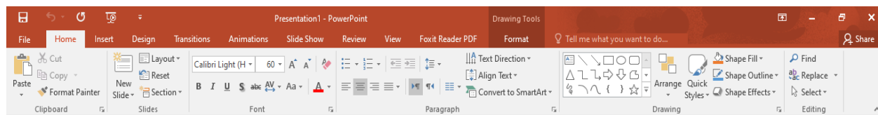
تصویر ۵: ریبن
