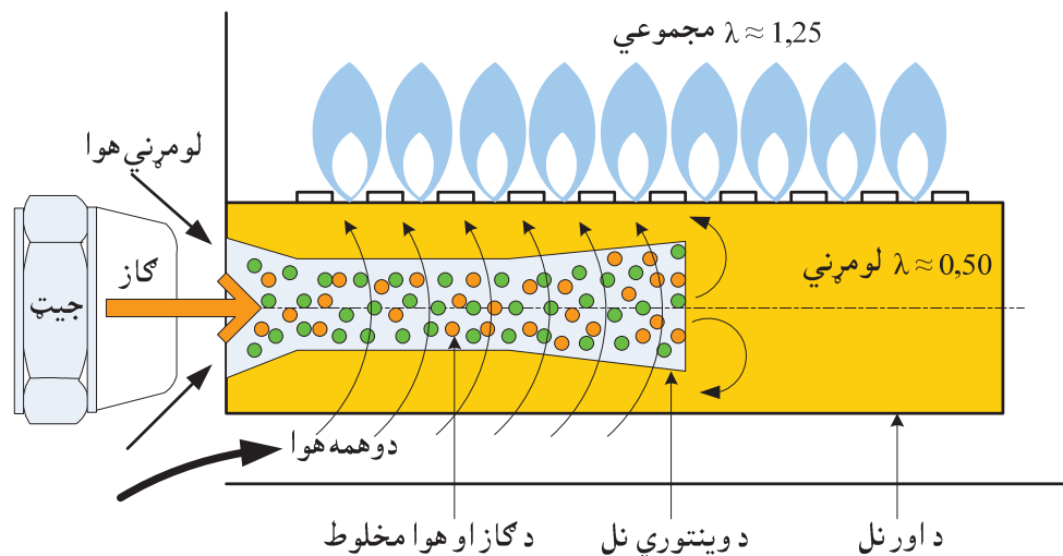
د گاز او هوا د نیمه گډولو برنر د کار پرنسیپ 49- شکل
