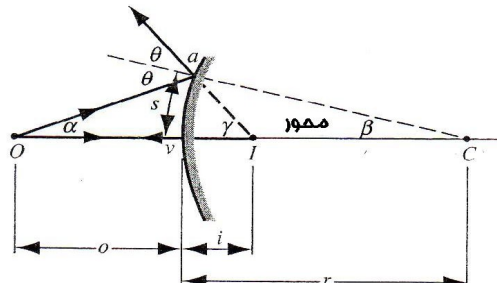
شکل ۲ - ۵ آئینه محدب تشکیل می‌دهد. این شکل را با شکل ۲ - ۱۴ مقایسه نماید.
