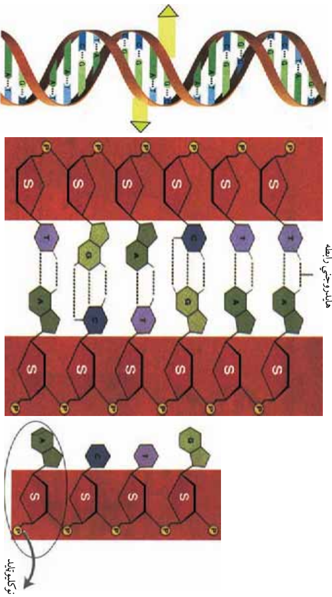
(۲-۳) شکل: د تازي شوي پروی په څنډ د DNA جوړښت
