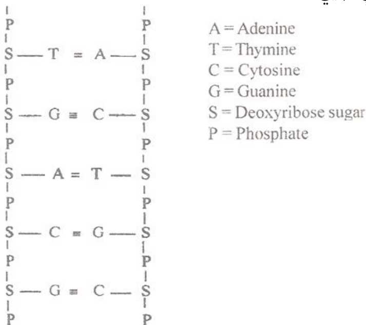
6-8 شکل: د DNA د مالیکولونو برخې رانښيي. د پیورینو او پیریمیدینو ترمنځ هایډروجنی رابطې وجود لري د آډنین او تایمین (A=T) ترمنځ دوه ګوني هایډروجنی رابطه وجود لري او د
