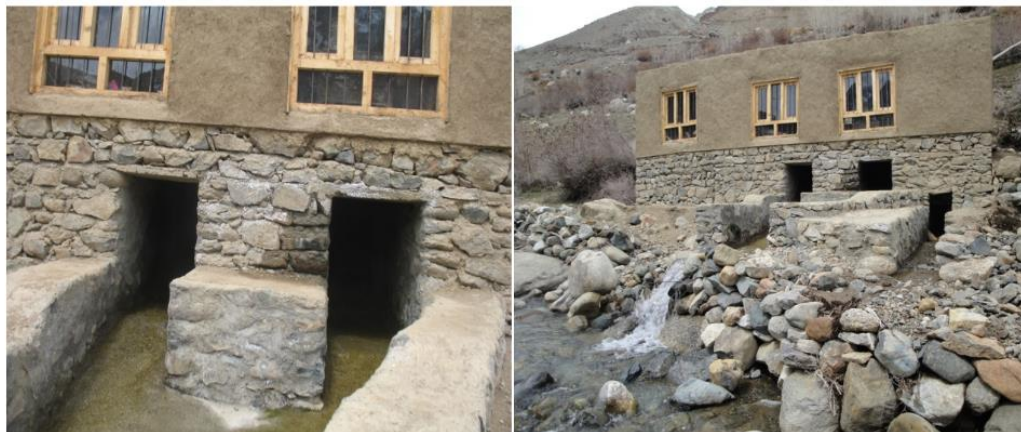
Tailrace canal
