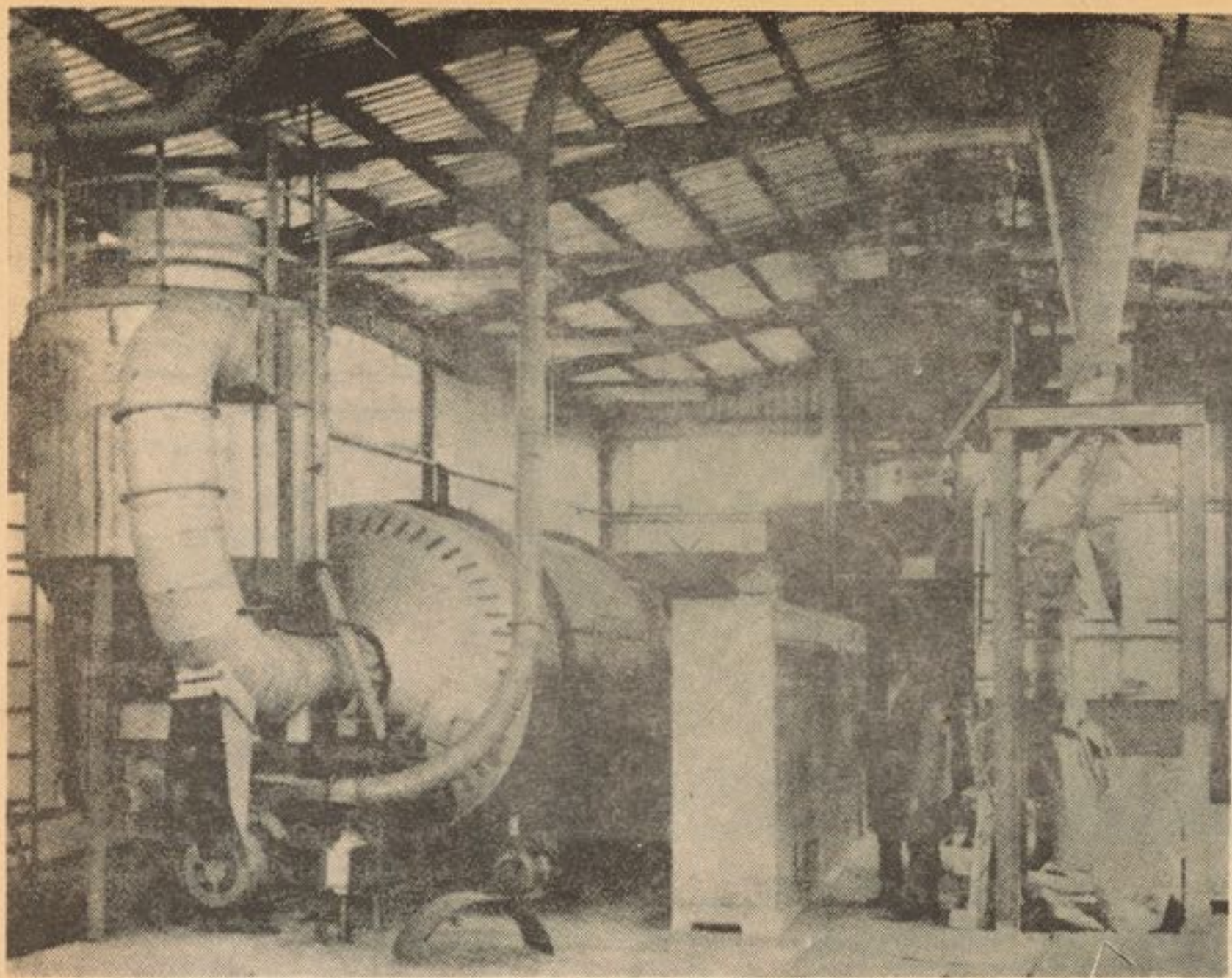
این دستگاه تصفیه جدیدترین دستگاهی است که قدرت تولید زیاد شکر را دارد.
