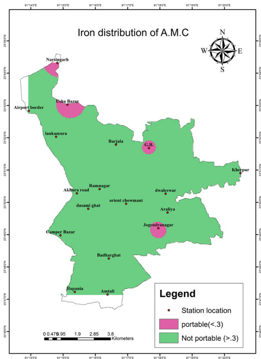
Fig. 2 Iron map
