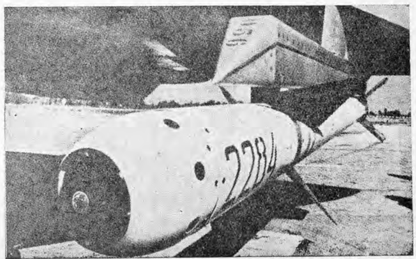
داسرائیلو شافریر ډوله راکت
