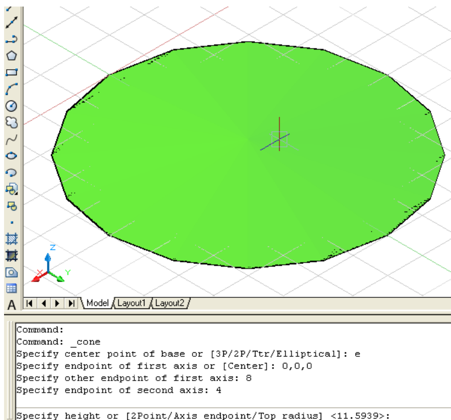
شکل د (۳۸-۱) Modeling) منیو څخه د مخروط (Cone) په هدایت کې د کار د شروع د مخه د لاندې سطحه رسمول د (E) لږویه او د محور و انتخاب
