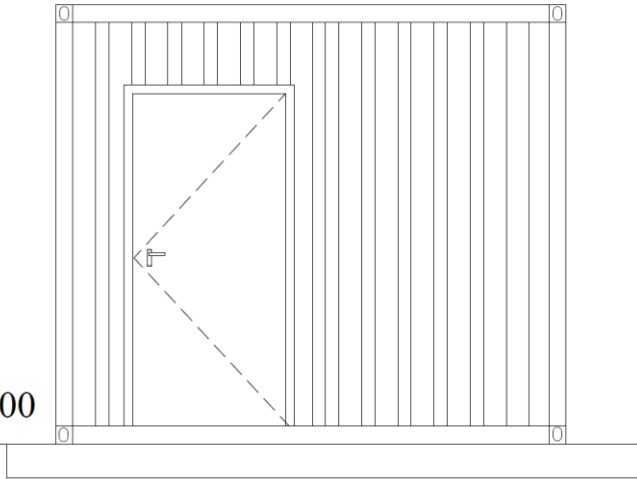
نمای پیشروی کانتینر تشناب مردانه و زنانه تی آی ام
