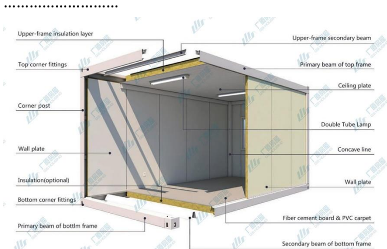
نمای سه بعدی تشریح کانتینر فلت پک
