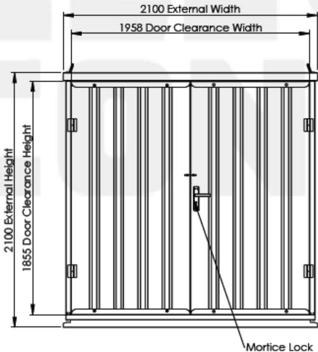
نمای دروازه کانتینر فلت پک ۵ در ۲ متر
