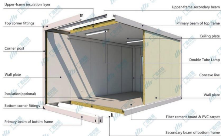
نمای سه بعدی تشریح کانتینر فلت پک
