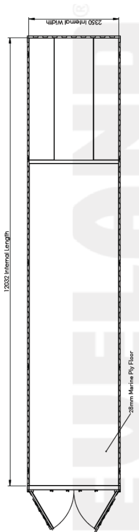
پلان کانتینر ۴۰ فوت ستندرد
