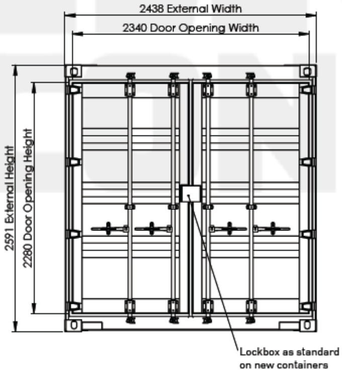
نمای دروازه کانتینر ۲۰ فوت استاندارد
