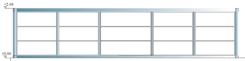
د تی آی ام حمامونو لرونکي كانتینر دپوال اسکلپت بندی پلان
