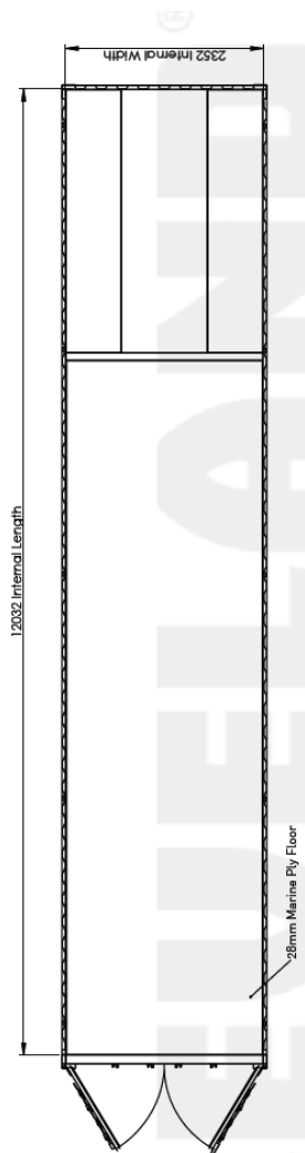
۴۰.۱۶ فته اوچت کانتینر پلان
