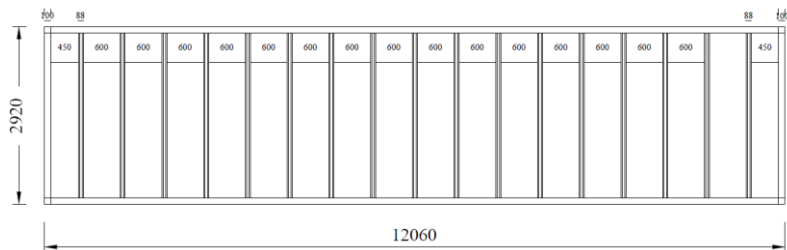
د تی آی ام حمامونو لرونکي كانتینر د غولي اسکلپت بندی پلان
